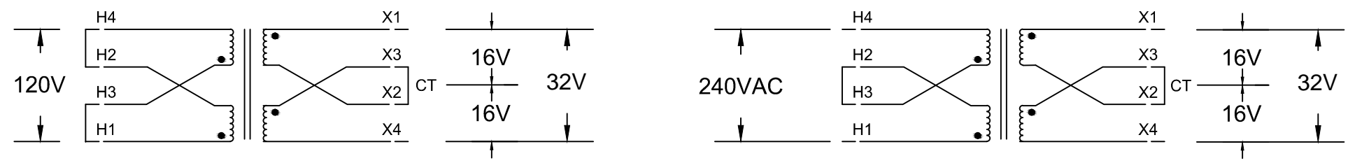
120VAC WIRING
